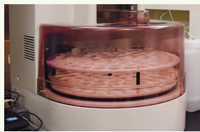
全有機炭素測定装置
